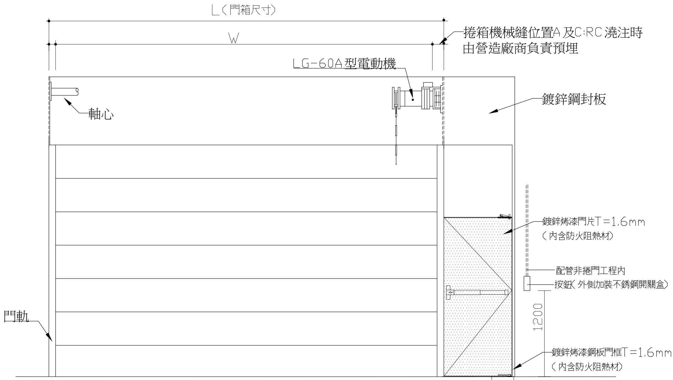
立 面 圖
