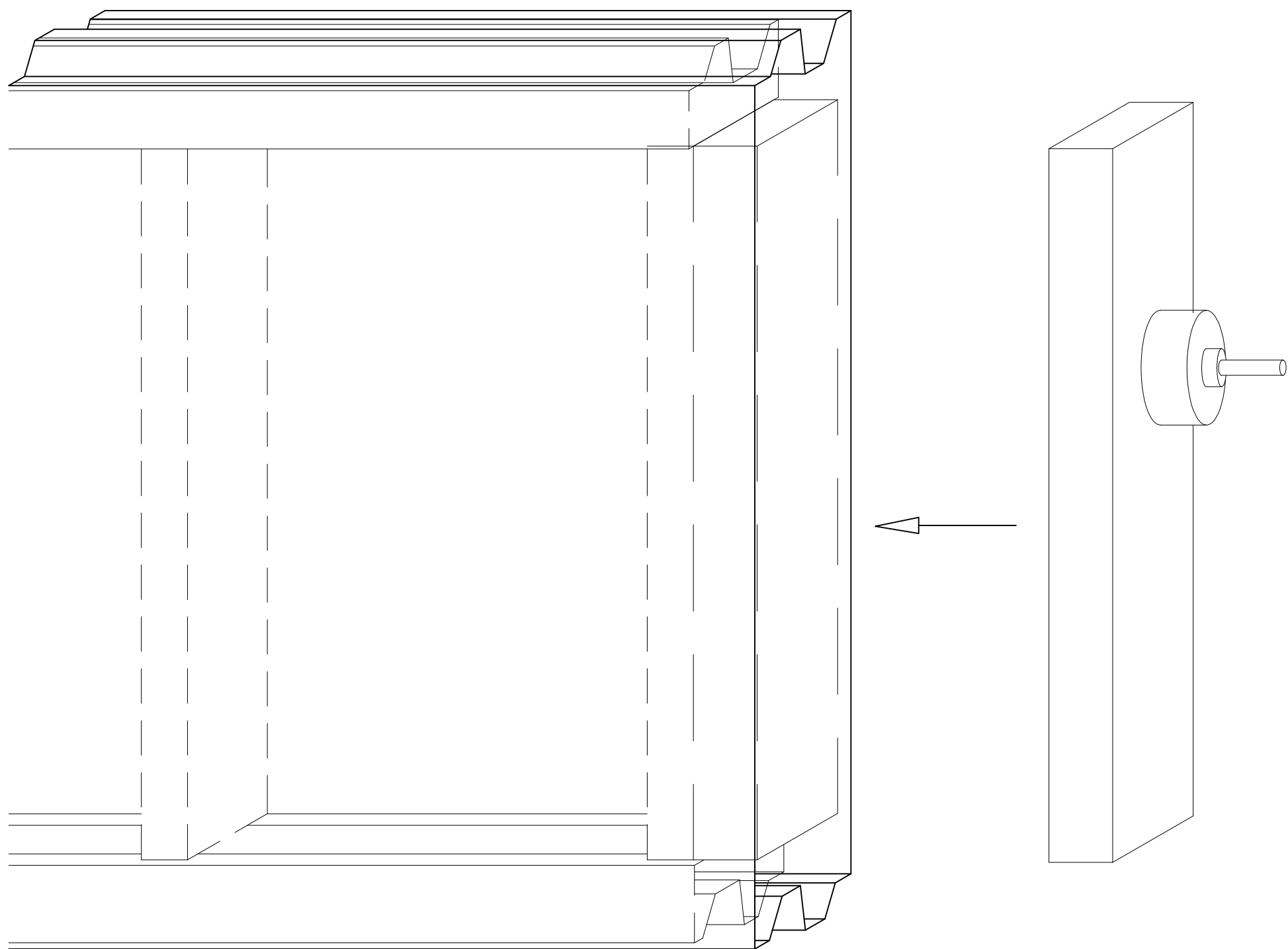
快速維修拆卸圖示
